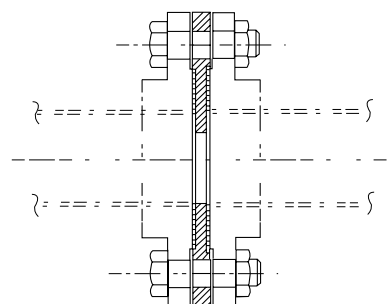
▶ Perturbateur type "Obturation partielle de section"
